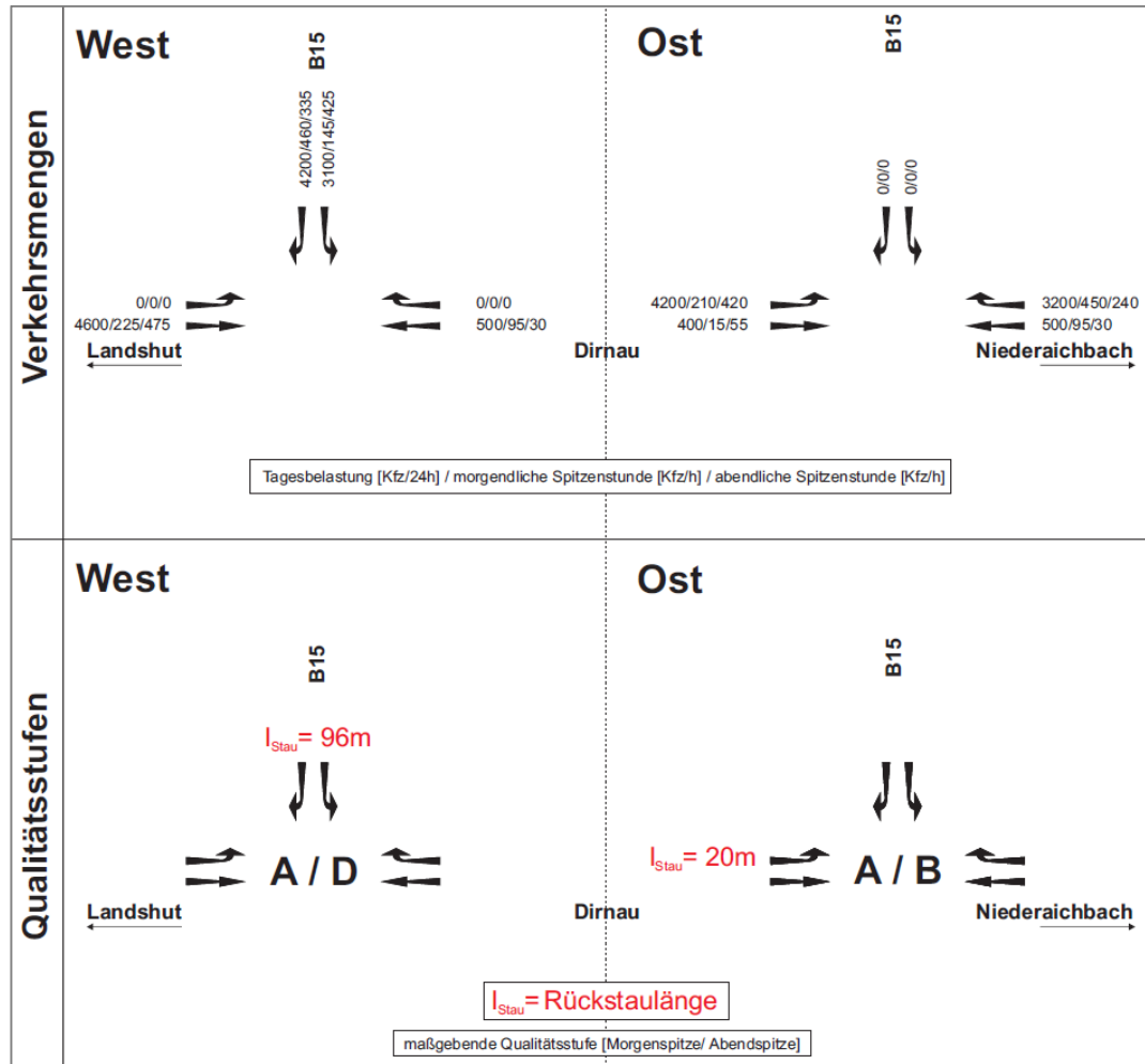
Abbildung 14: Knoten Dirschau – Leistungsfähigkeitsnachweis nach HBS 2015
