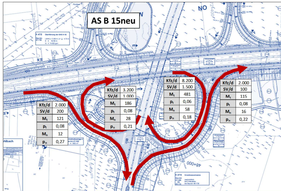
Abbildung 12: Lärmkennwerte 2035 am Kreuz Landshut für die südlich der A 92 gelegenen Knotenpunktarme
