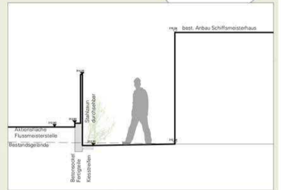
Querschnitt (A-A') Einfriedung M: 1:50
